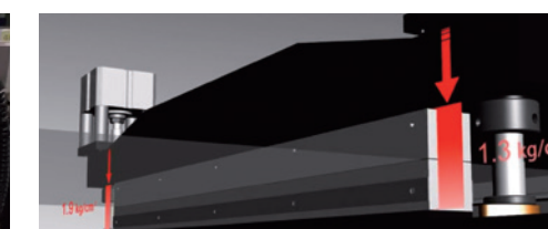
熱封座氣壓調整裝置 (獨立式)
